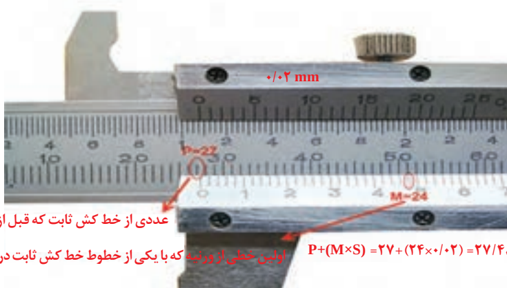
شکل ۱-۲۳- قرائت کولیس
