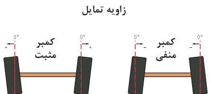
شکل ۴۴- ۳- زاویه تمایل
