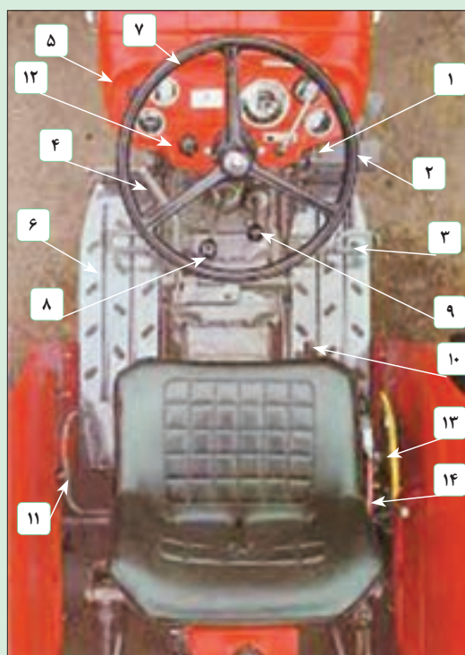
شکل ۲-۴- اجزای هدایت و کنترل تراکتور MF۲۸۵
