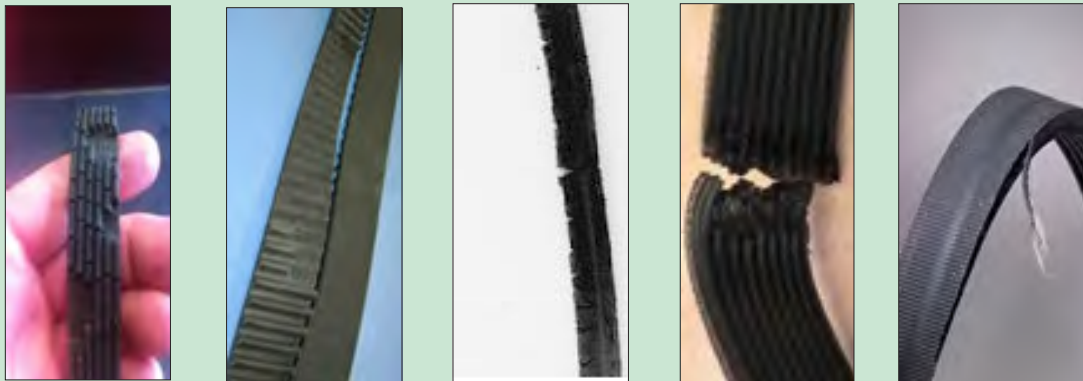
شکل ۶۵-۵- خرابی انواع تسمه
