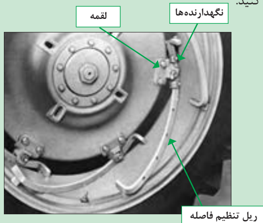
شکل ۳۵-۵- رینگ ریلی
