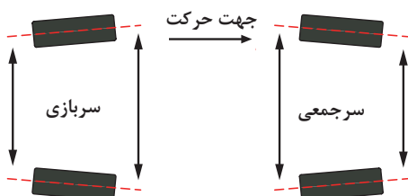
شکل ۴۵- ۳- زاویه سرجمی
