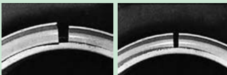
شکل ۳۲- ۵- ب - اتصال صحیح بغل رینگ
