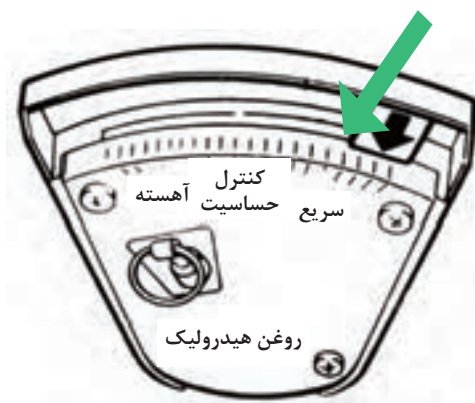
شکل ۲۵-۴ اهرم کنترل حساسیت
