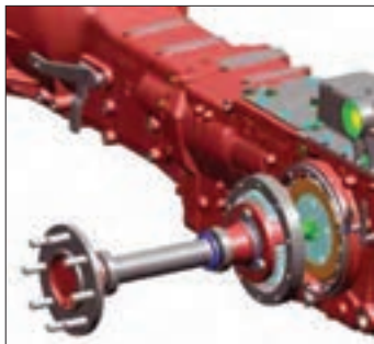
شکل ۲۳- ۳- کاهنده نهایی
