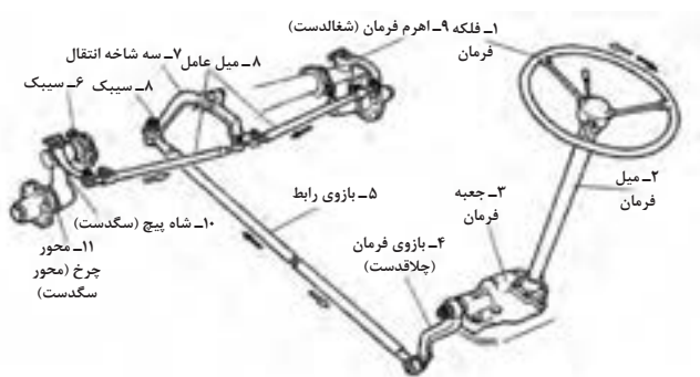
شکل ۳-۳۶ اجزای فرمان مکانیکی
