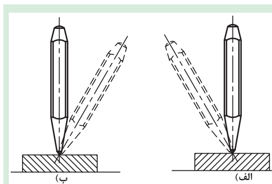
شکل ۳۱-۱- طرز صحیح قرار دادن سنجه نشان
